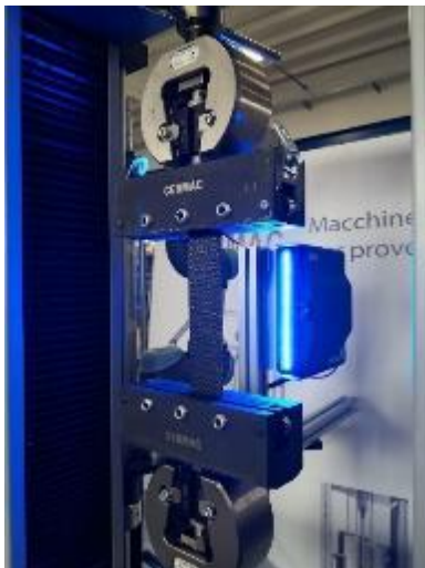
Video estensimetro M5
